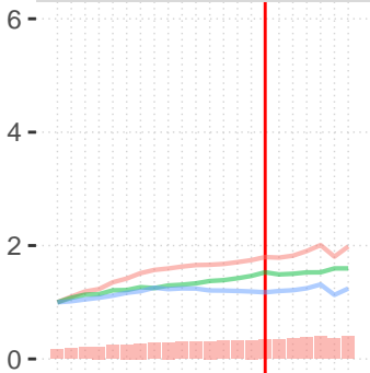
Other GI_AHRQ
